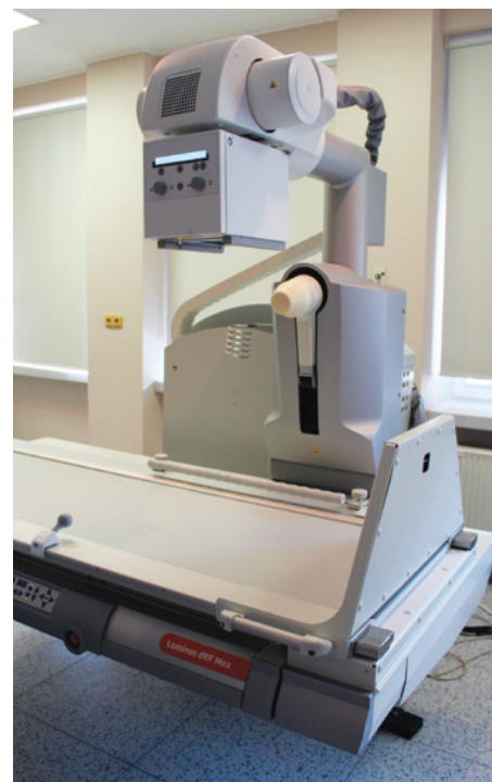
Skiaskopicko-skiagrafický RTG
